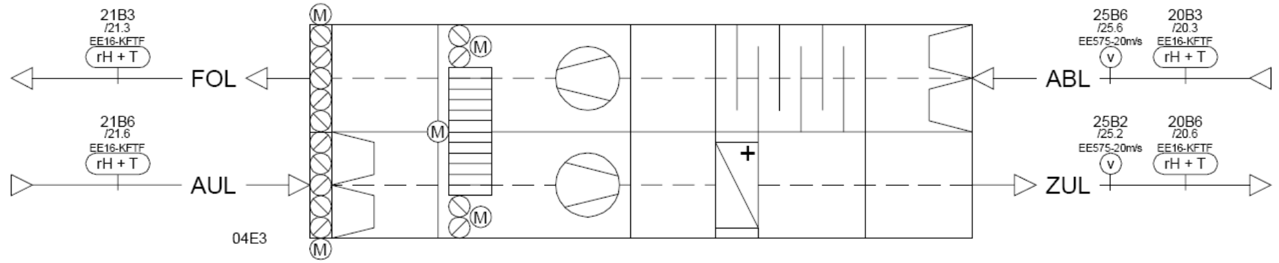
Lüftungsgerät
